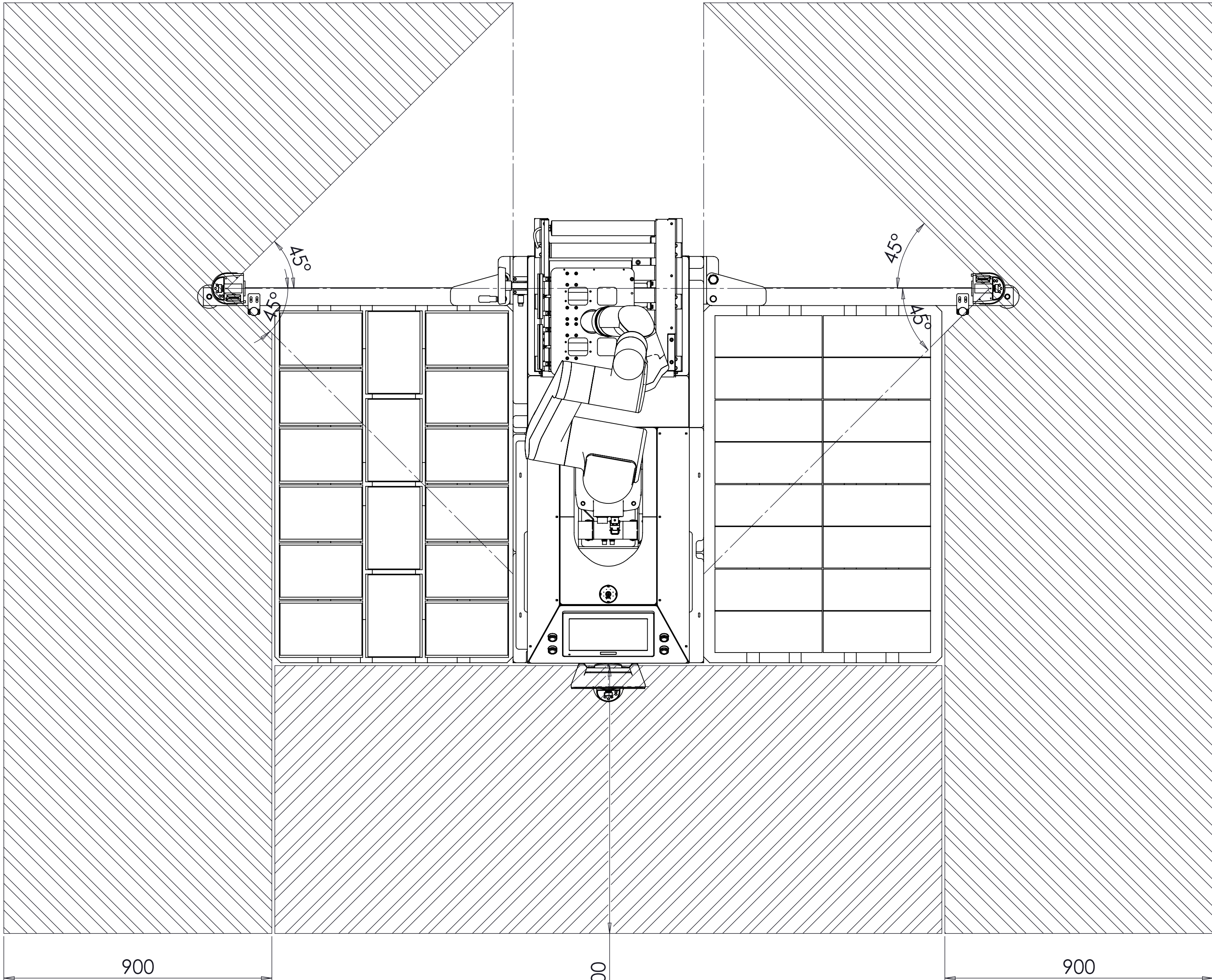
Area copertura scanner laser
