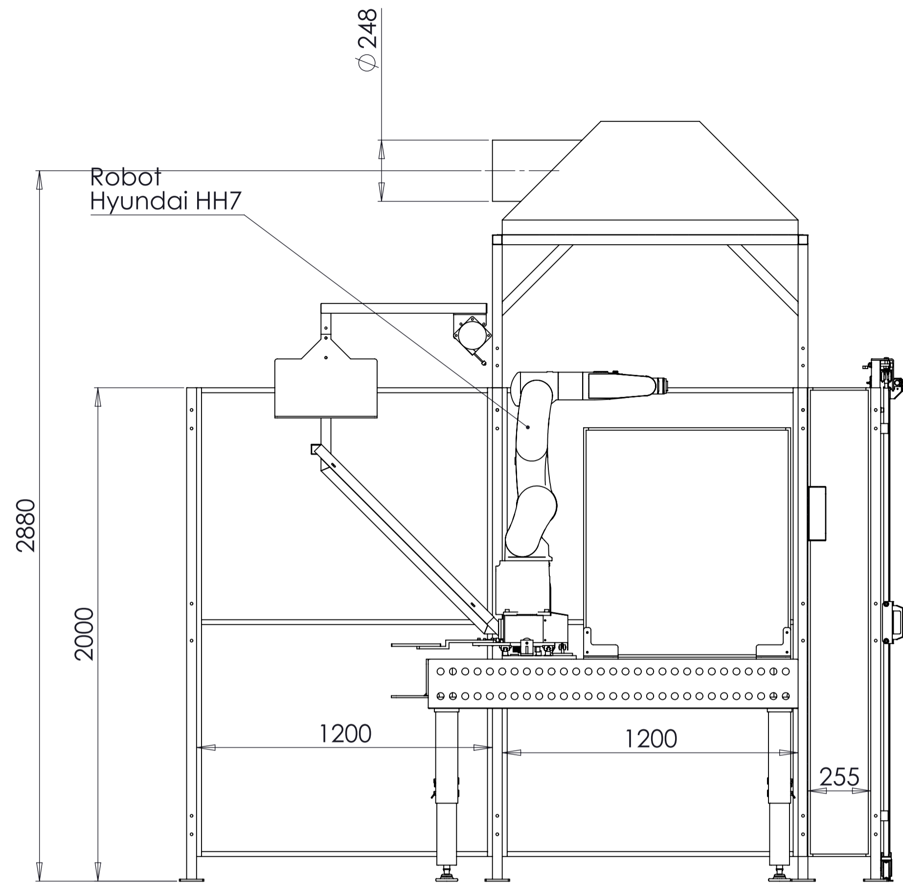
SEZIONE A-A
